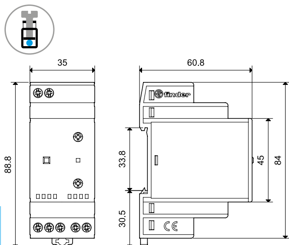
Typ 11.41 Schraubklemmen
