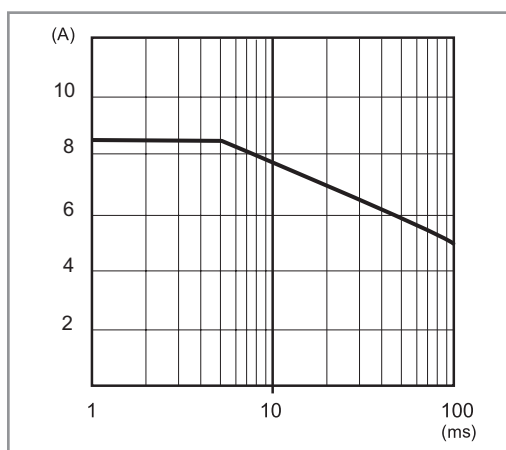
P78-6 Einschaltspitzenstrom-Belastbarkeit (78.61)
