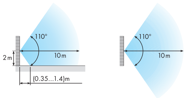
Senkrechter Erfassungsbereich
