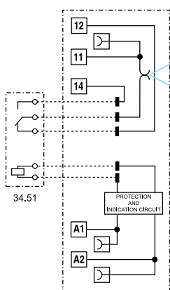
93.63 / 93.66
