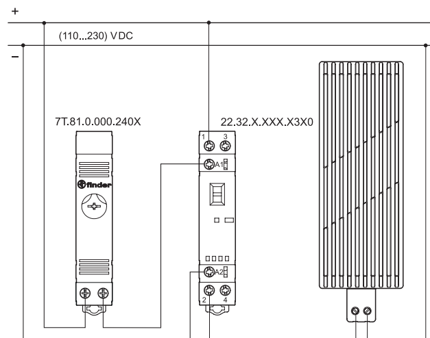
DC-Ausführung
