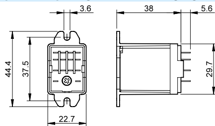
056.25 mit Relais
