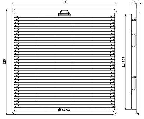
Typ 7F.02.0.000.5000
