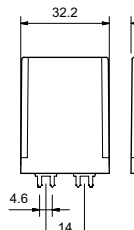
Typ 65.61-0300
