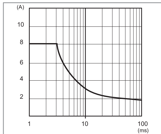
P78-3 Einschaltspitzenstrom-Belastbarkeit (78.36)
