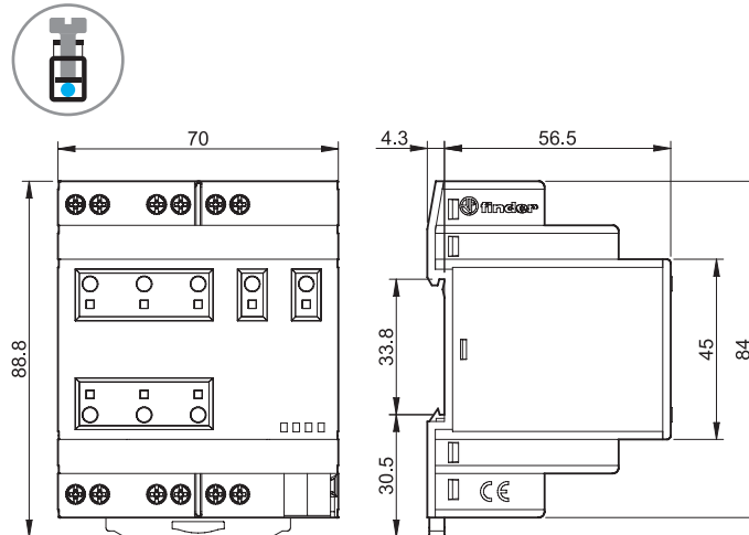
Typ 19.6K Schraubklemmen
