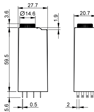
Typ 85.04
