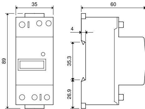
Typ 7E.16.8.230.0010
