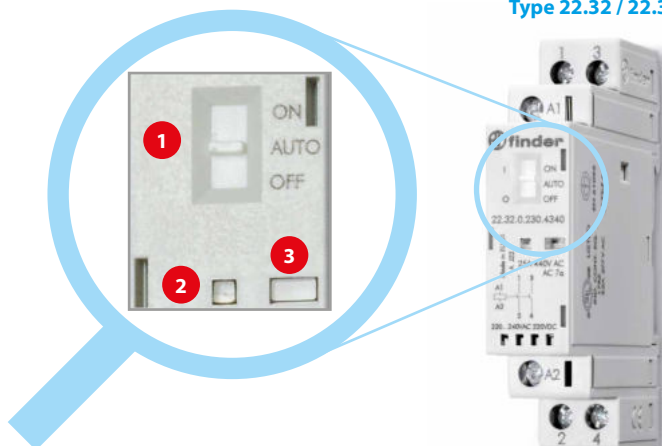
Typ 22.32 / 22.34
