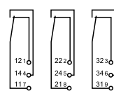
94.13
