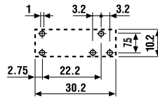
Ansicht auf die Anschlüsse
