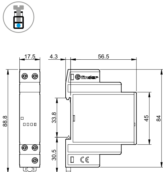
Typ 19.91 (Ausgangsmodul für 11.91) Schraubklemmen
