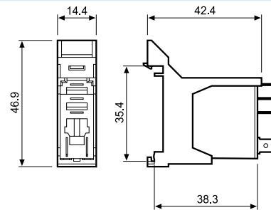
046.07 mit Relais
