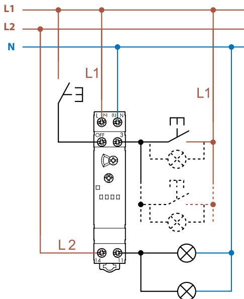
Typ 14.11 Treppenhaus-Lichtautomat und Last mit unterschiedlichen Phasen
