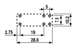
Ansicht auf die Anschlüsse
