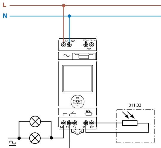
Typ 11.91
