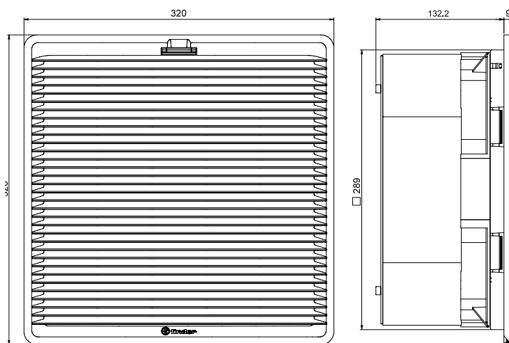
Typ 7F.20.x.xxx.5700
