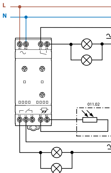
Typ 11.42
