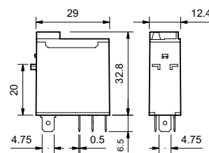
Typ 46.61
