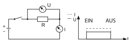
Strom-/Spannungsverlauf beim Schalten einer ohm'schen Last Abb.1
