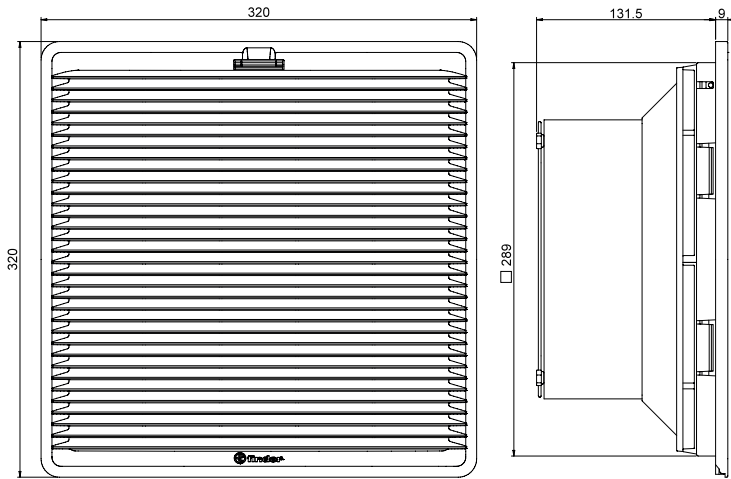
Typ 7F.20.x.xxx.5700
