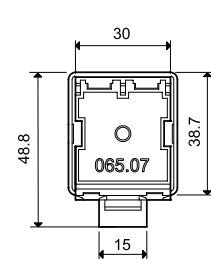
065.07
