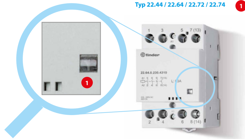
Typ 22.44 / 22.64 / 22.72 / 22.74
