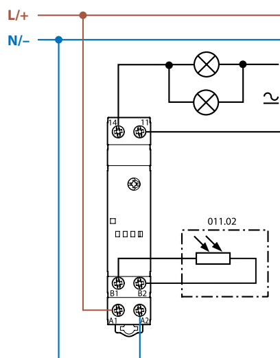
Typ 11.42
