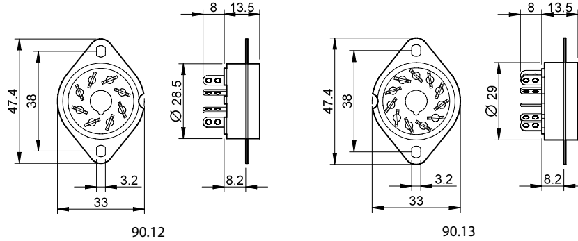
90.12
