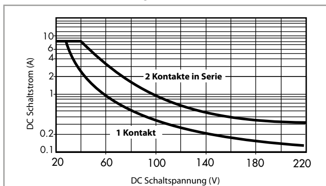
RR - Gleichstromschaltvermögen bei DC1
