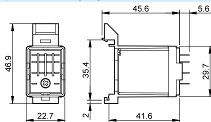
056.27 mit Relais
