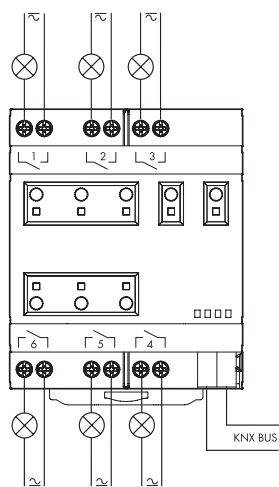
Typ 19.6K
