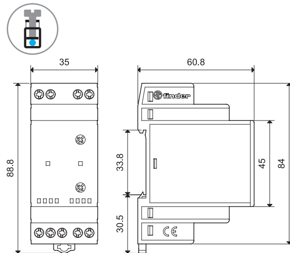
Typ 72.42 Schraubklemmen
